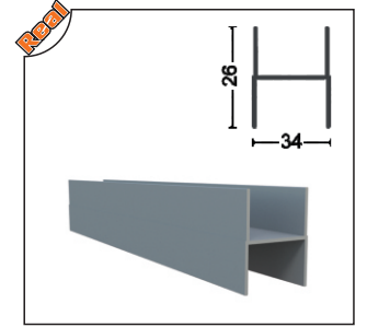
YNSRM-1009 Birleştirme Adaptörü Joining Adapter
